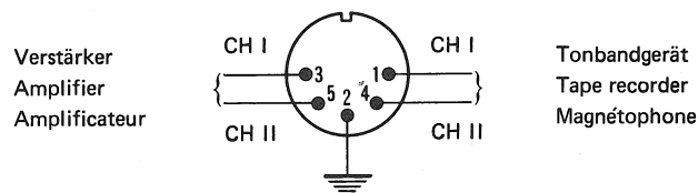
Sicht auf Stecker, Seite Lötflächen View on plug, solder lug side Vue de la fiche côté soudures
